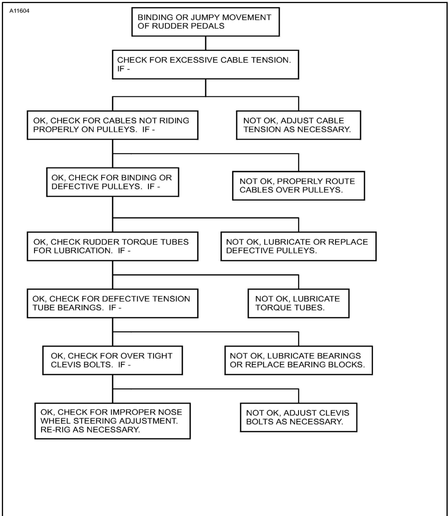
Figura 101: Folha 1: Tabela de solução de problemas do sistema de leme
